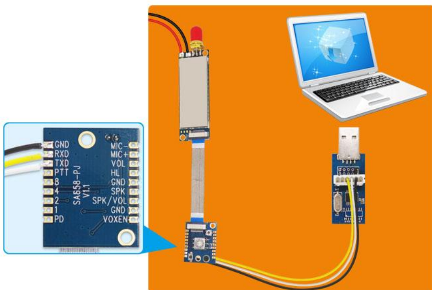
对讲模块TTL接口连接示意图
